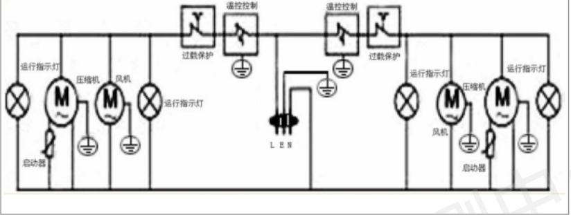
电气原理图
