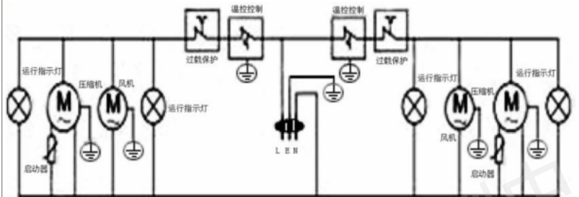
电气原理图
